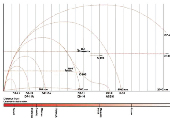
Rys. 2. Zasięg oddziaływania chińskich sił strategicznych w regionie Morza Południowochińskiego i wysp zachodniej części Oceanu Spokojnego Źródło: Military And Security... , 2013
